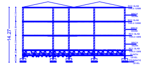
SECTION A-B
